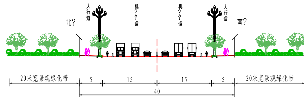
南新大道道路标准横断面图
